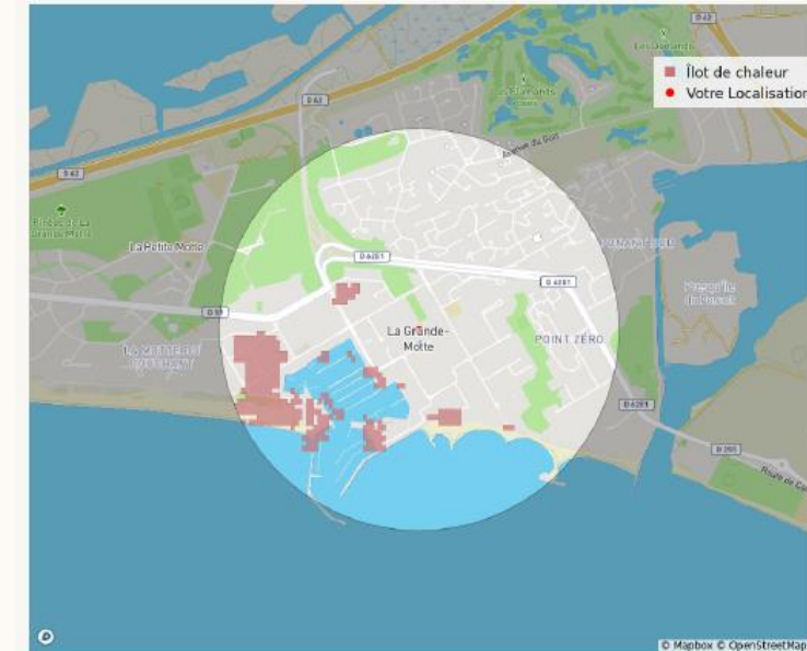
Carte des îlots de chaleur dans la commune
