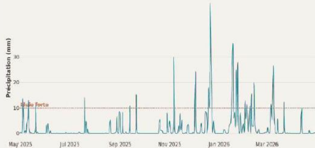
Graphique des précipitations sur l'année glissante
